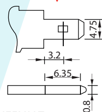
КЛЕММ T1
